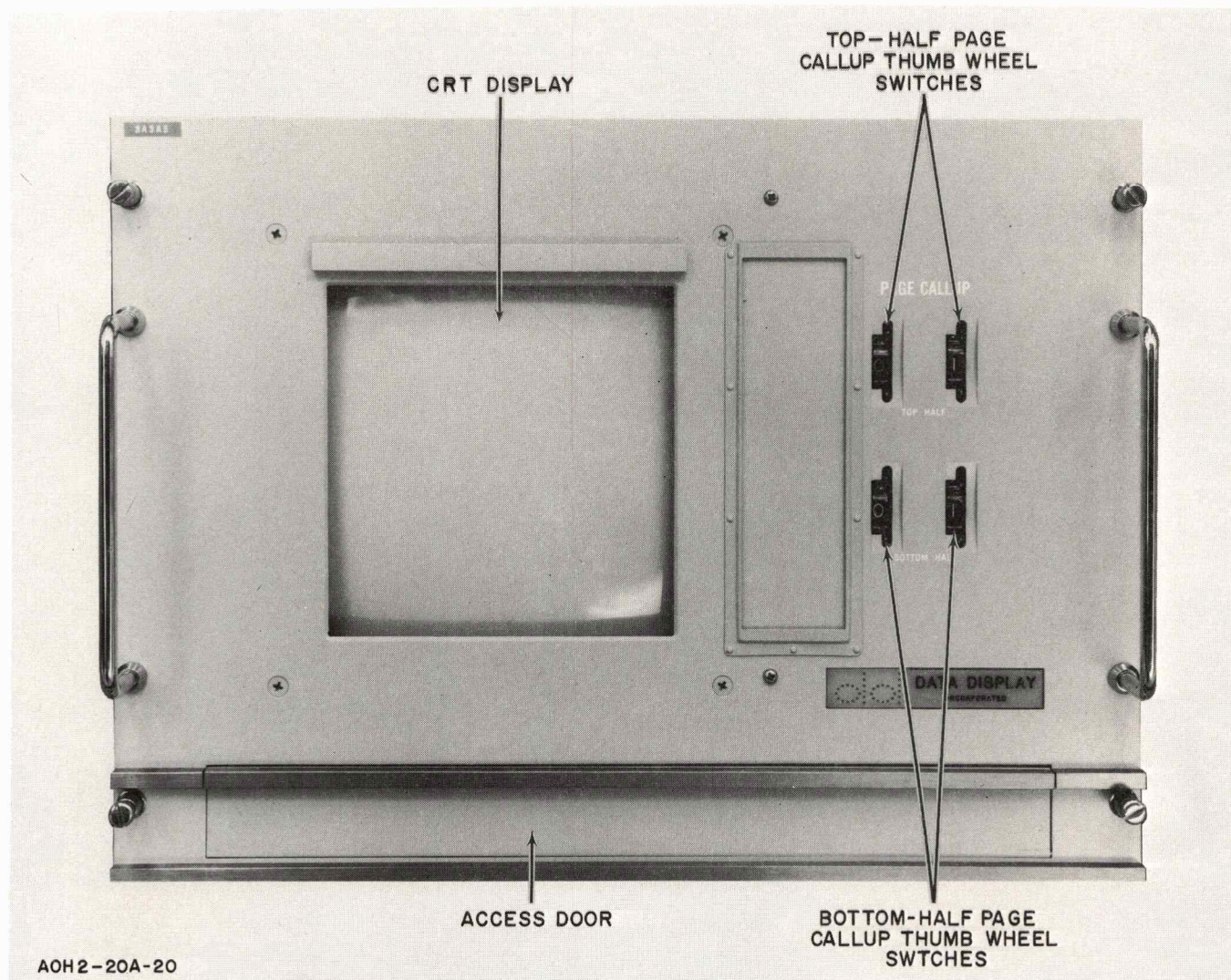
Figure 3-6. CRT Module
