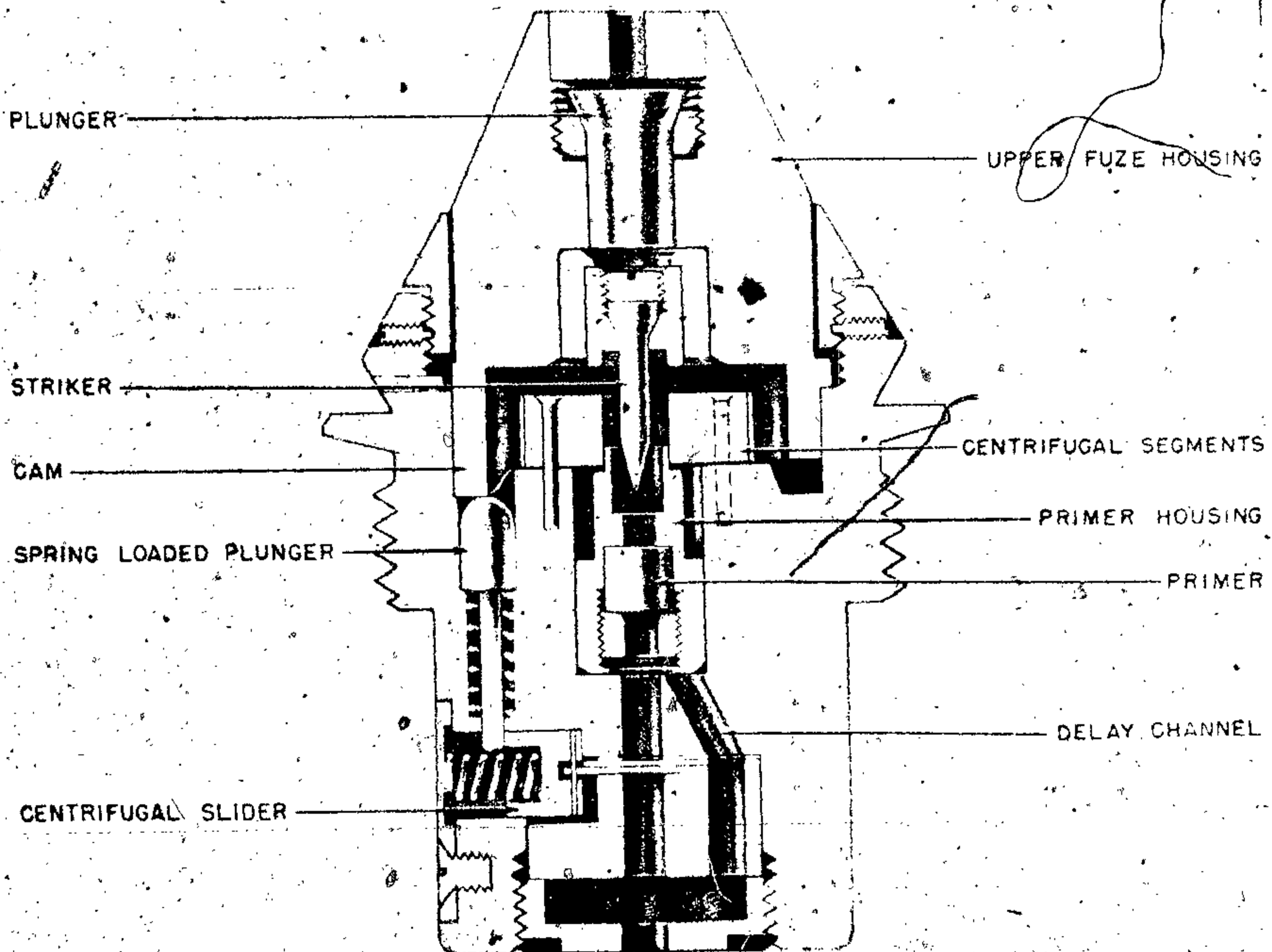
Figure 585—Hbgr. Z. 35 D
