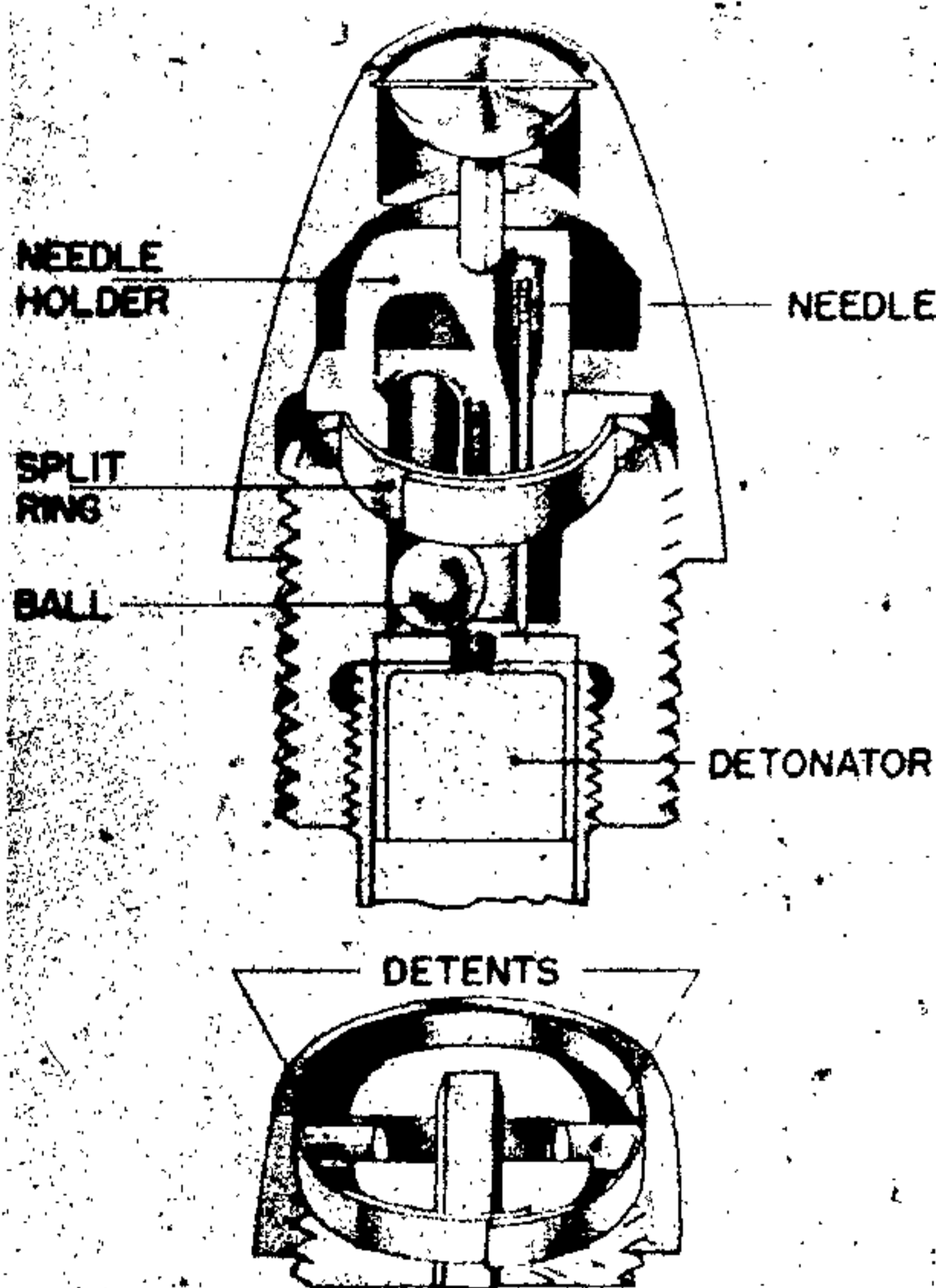
Figure 553—A. Z. 1503 and A. Z. 1504
