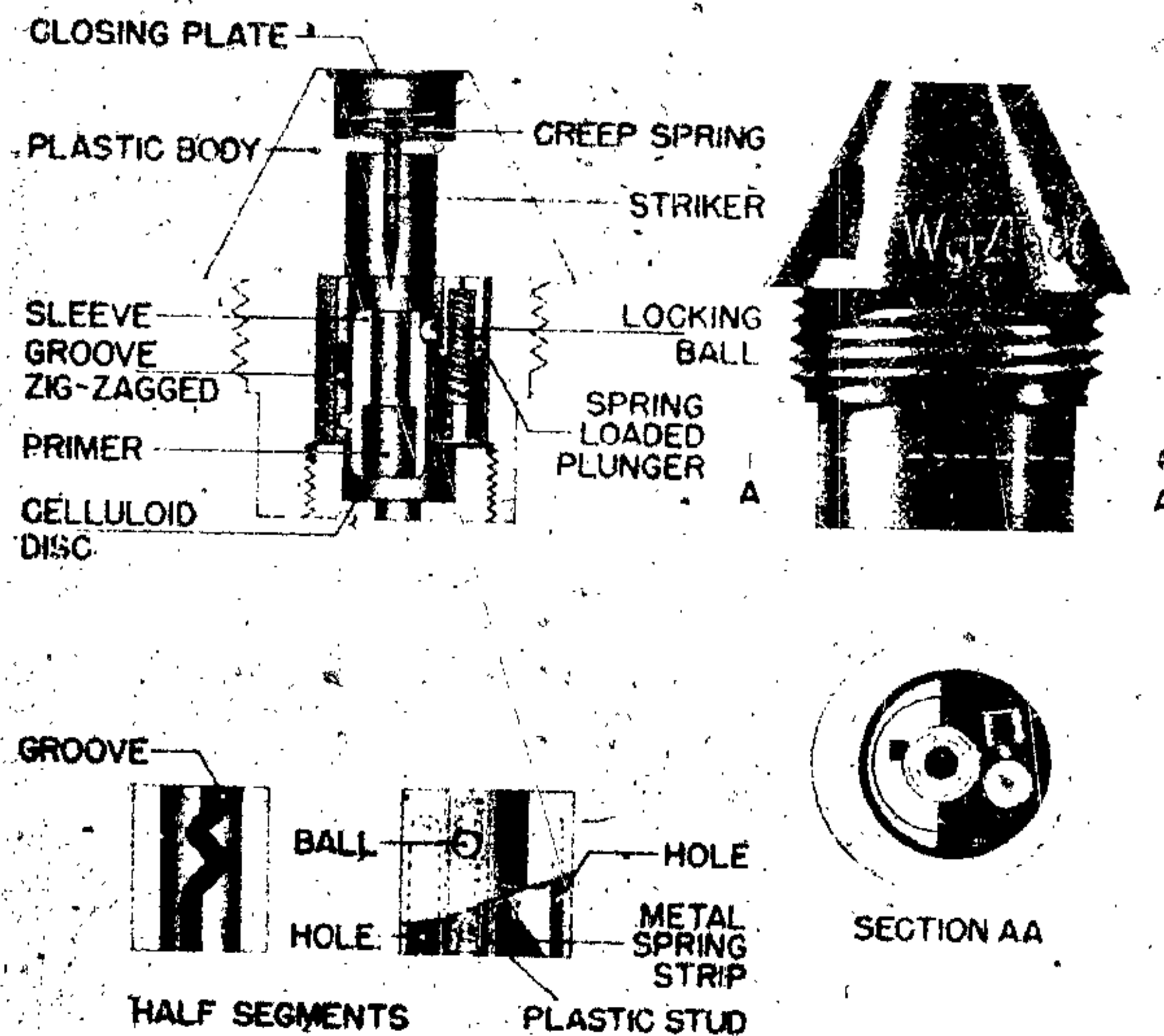
Figure 590—Wgr. ZT. acb
