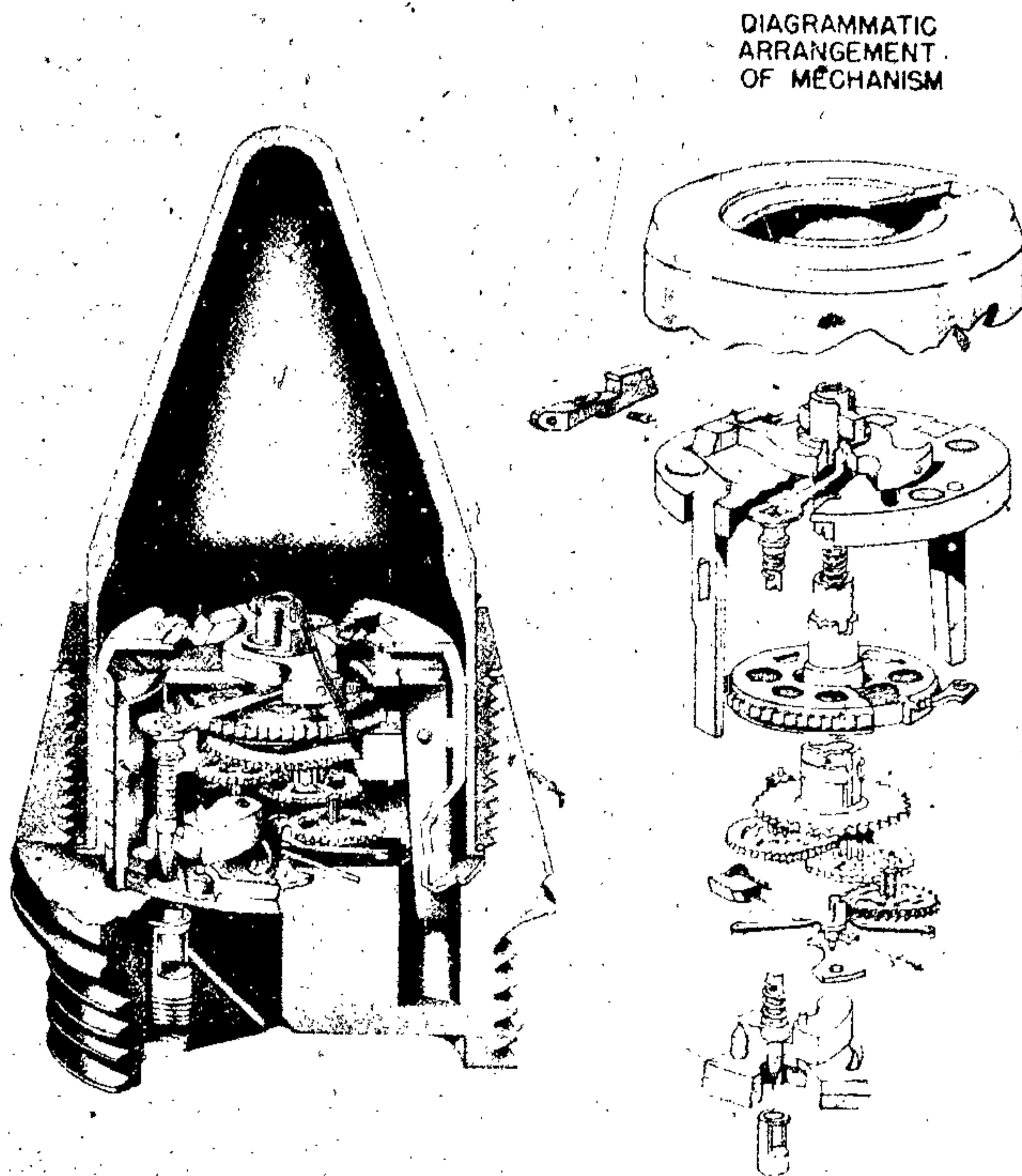
Figure 593A—Zt. Z. S/30
