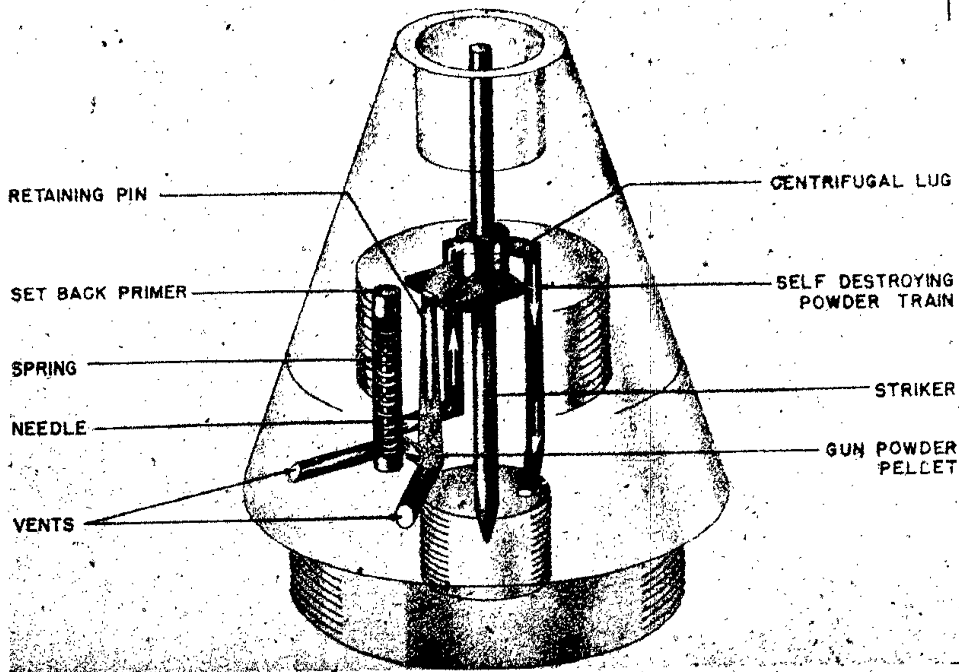
Figure 565—3.7-cm Kopfzunder Zerl. Pv.
