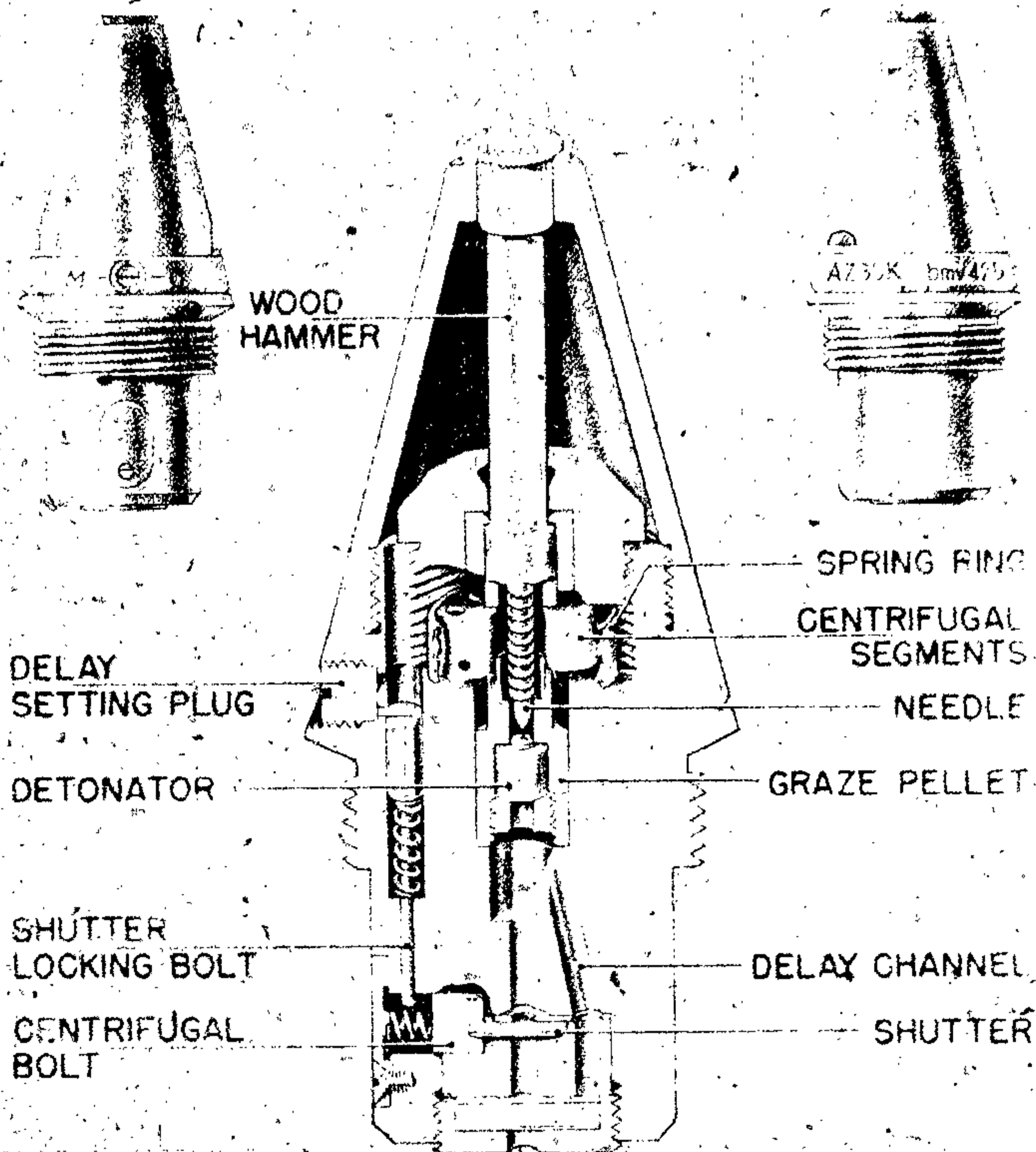
Figure 582—A. Z. 35 K
