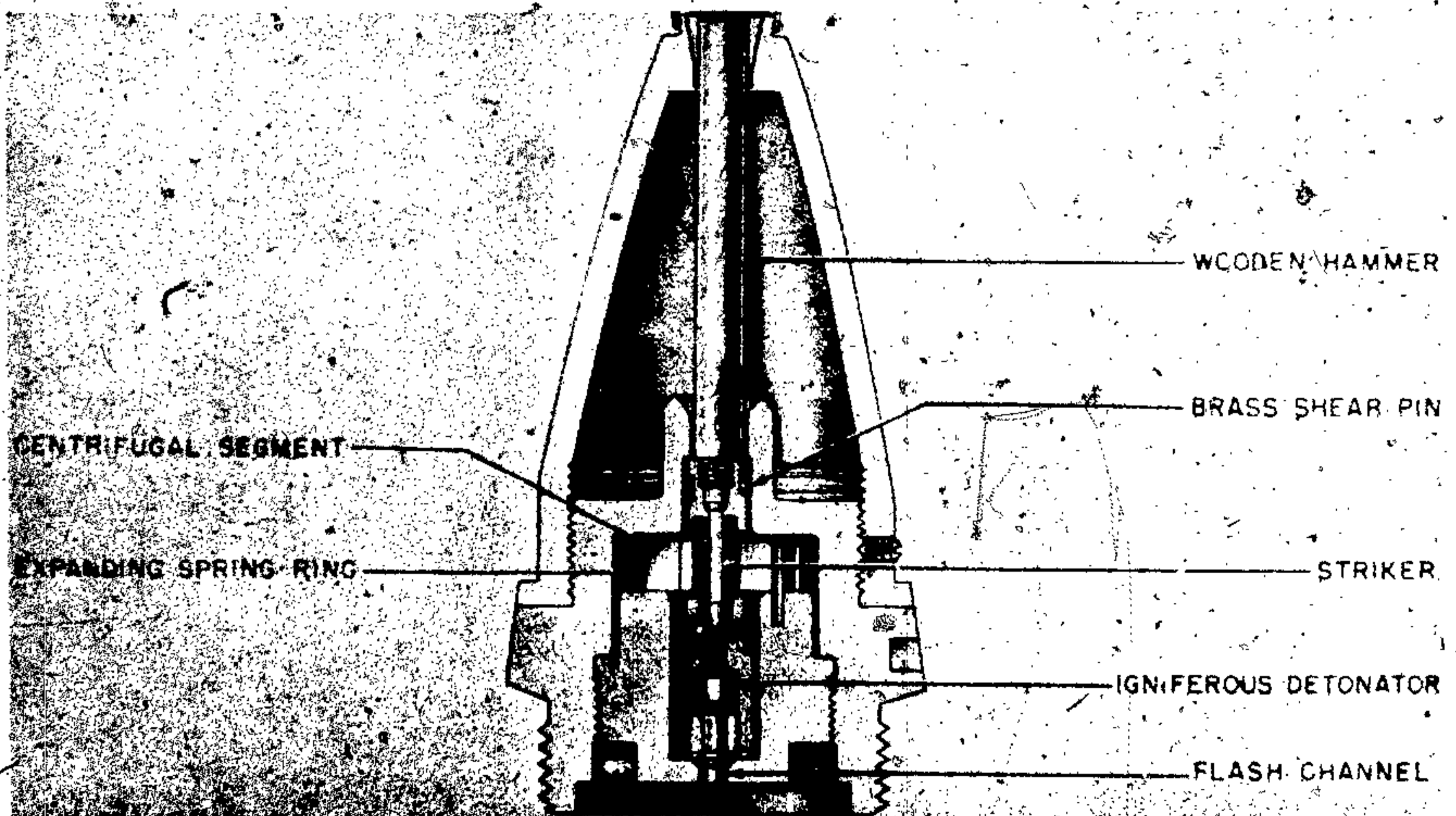
Figure 570—E. K. Zdr. C/28
