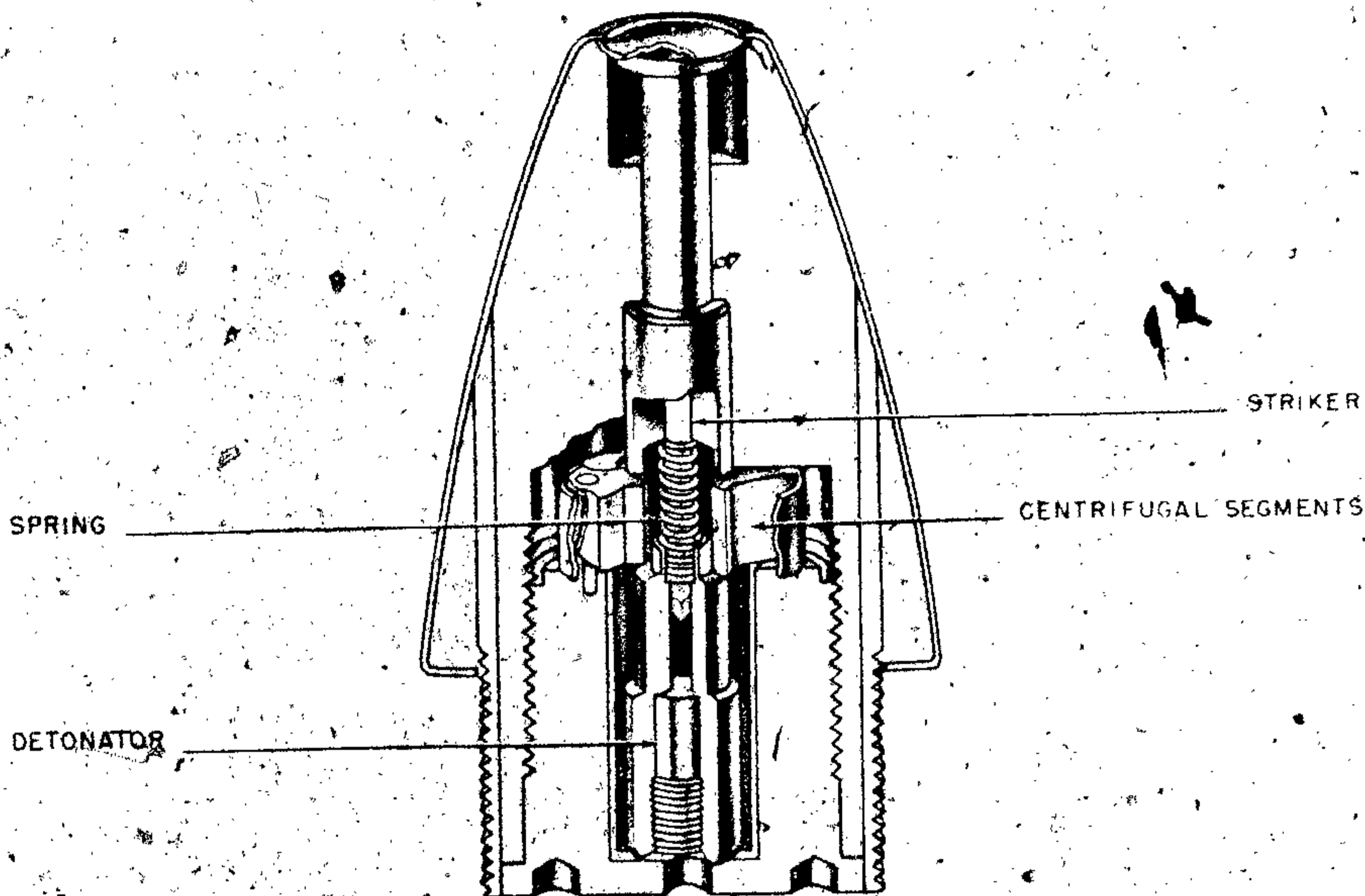
Figure 581A—Kl. A. Z. 23 Nb
