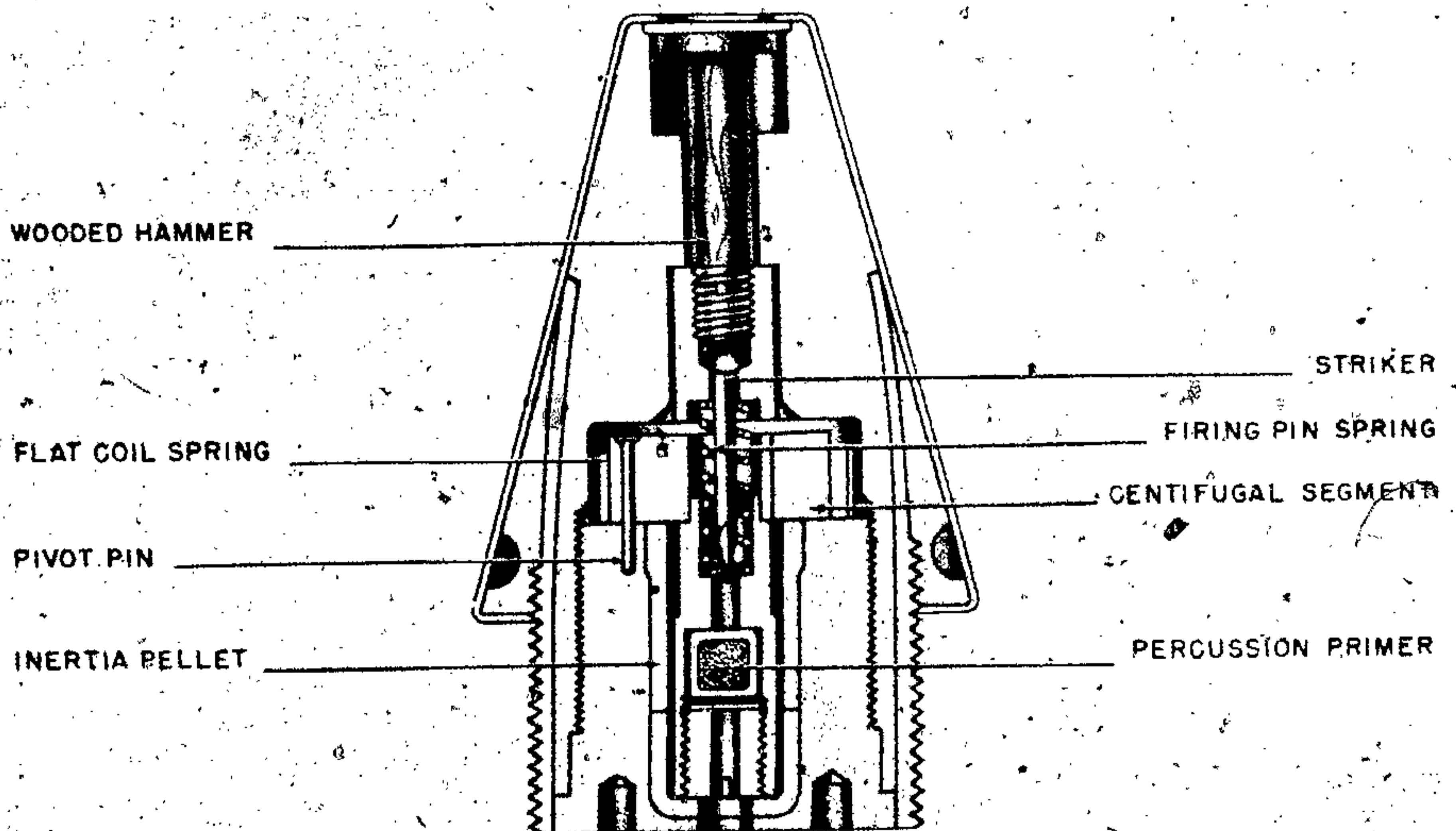
Figure 581C—Kl. A. Z. 40 Nb (Pr)
