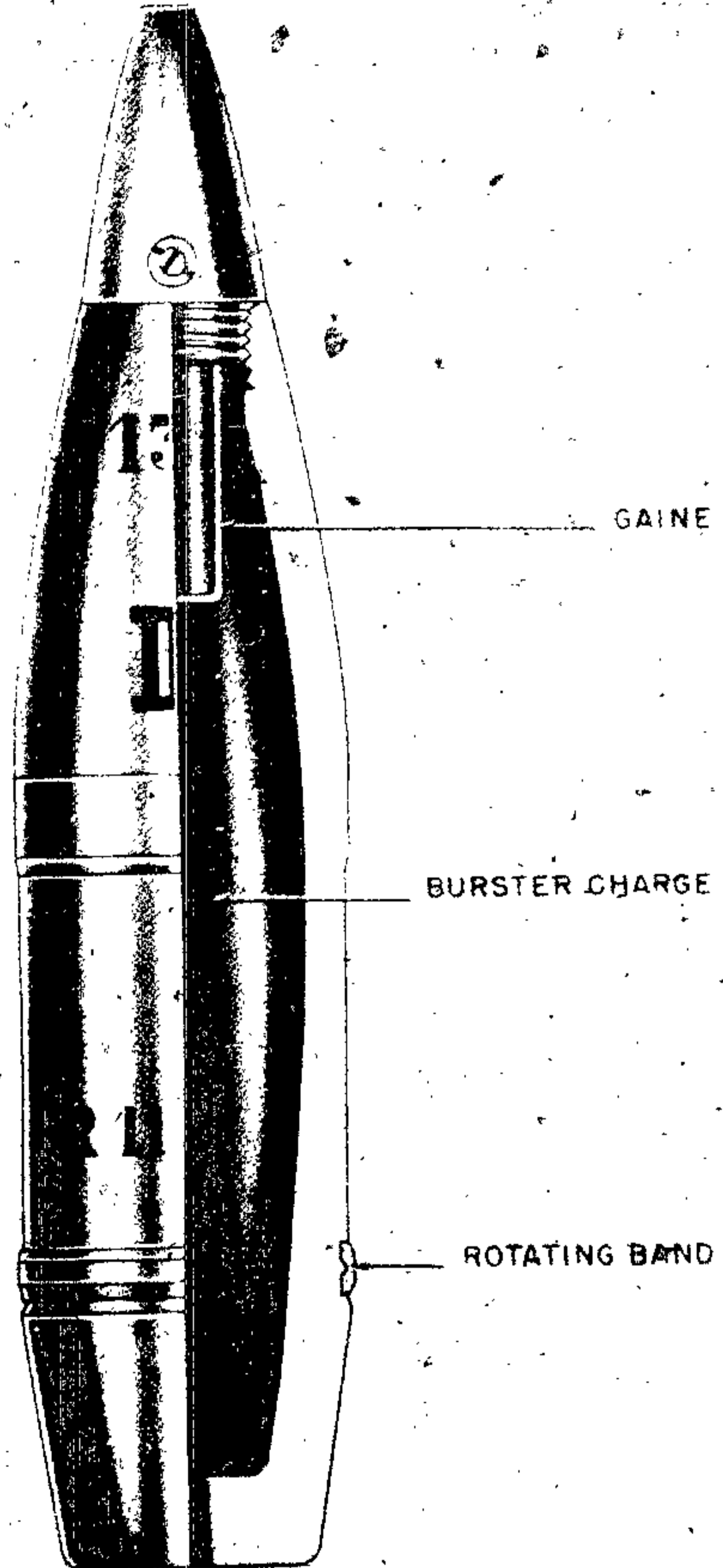
Figure 463—H. E. Projectile, 105-mm, 10.5-cm K. Spr. 38 (f)
