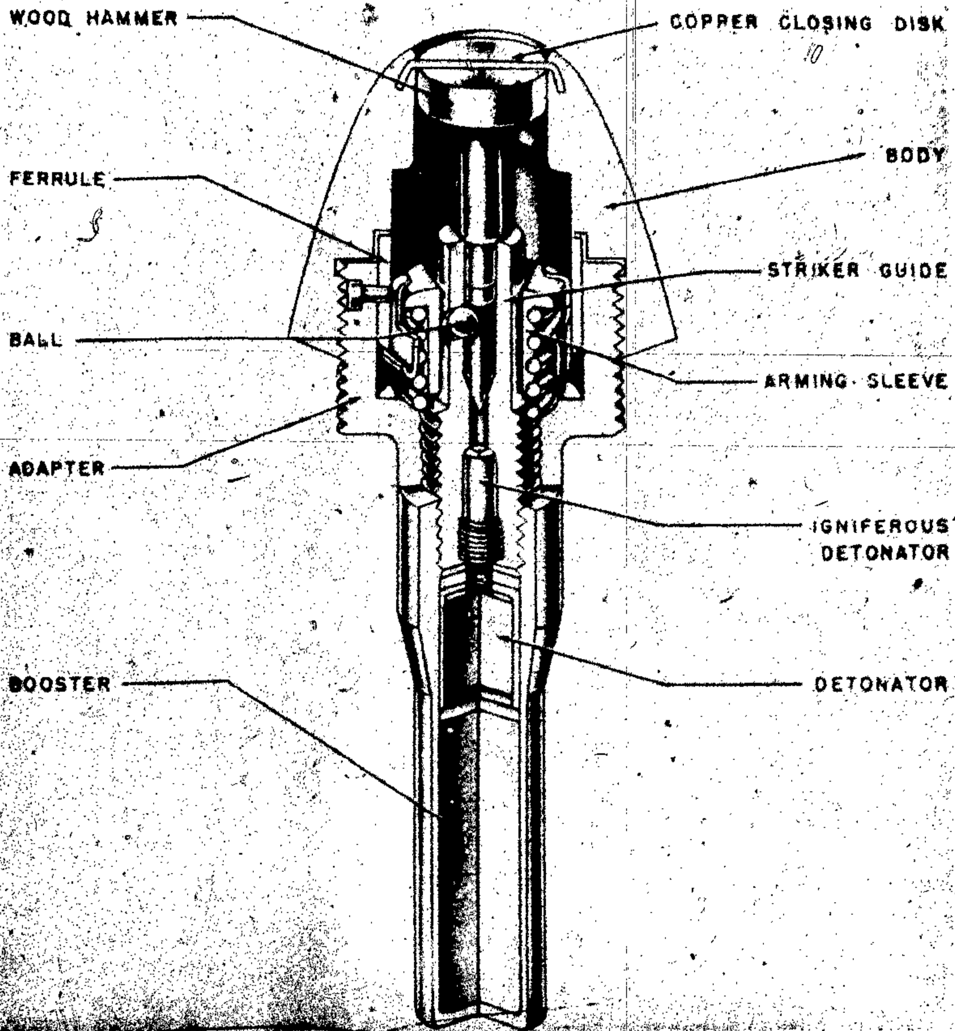
Figure 568—D. A. K. Z. 38
