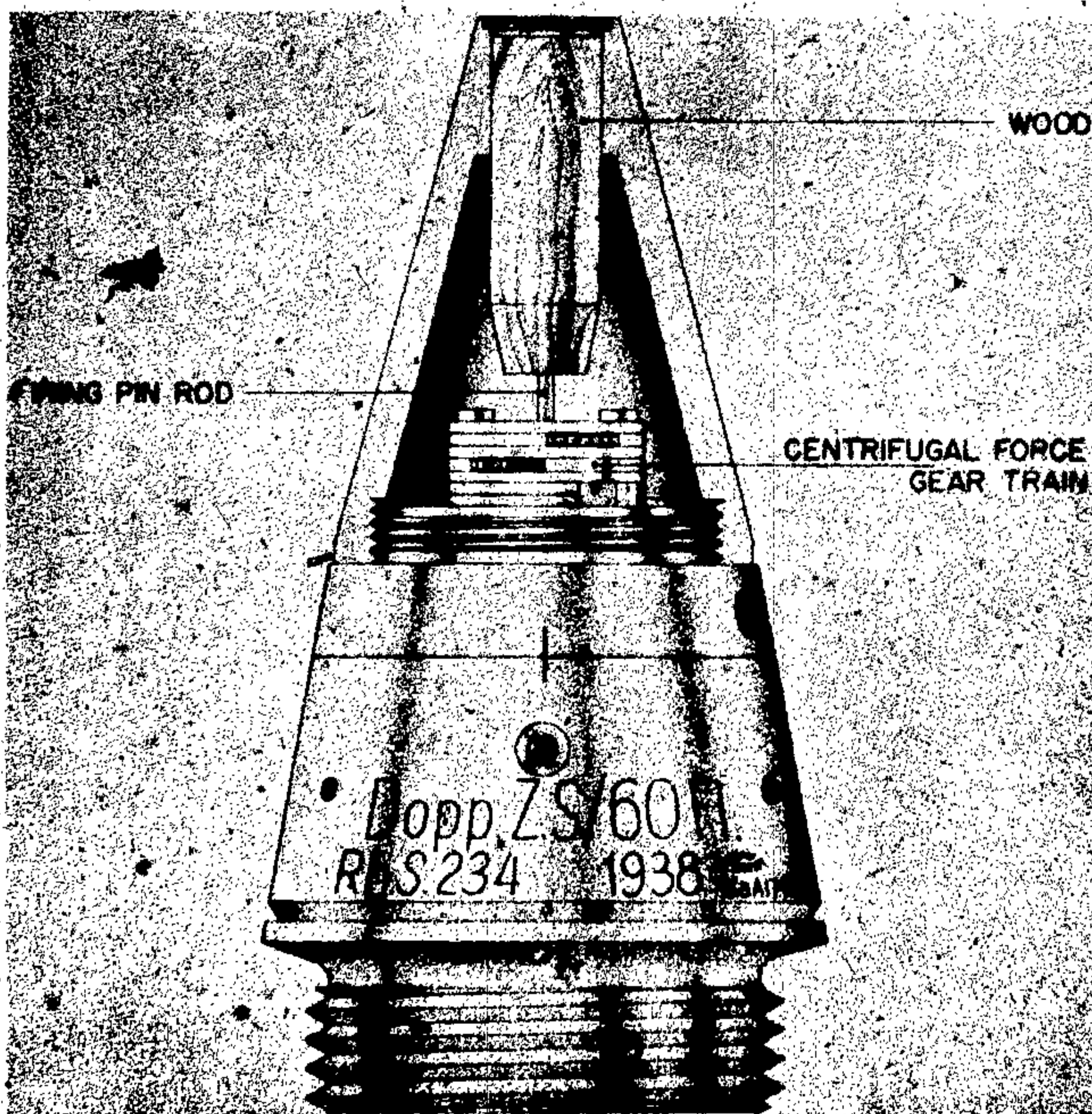
Figure 596—Dopp. Z. S/60 FI.
