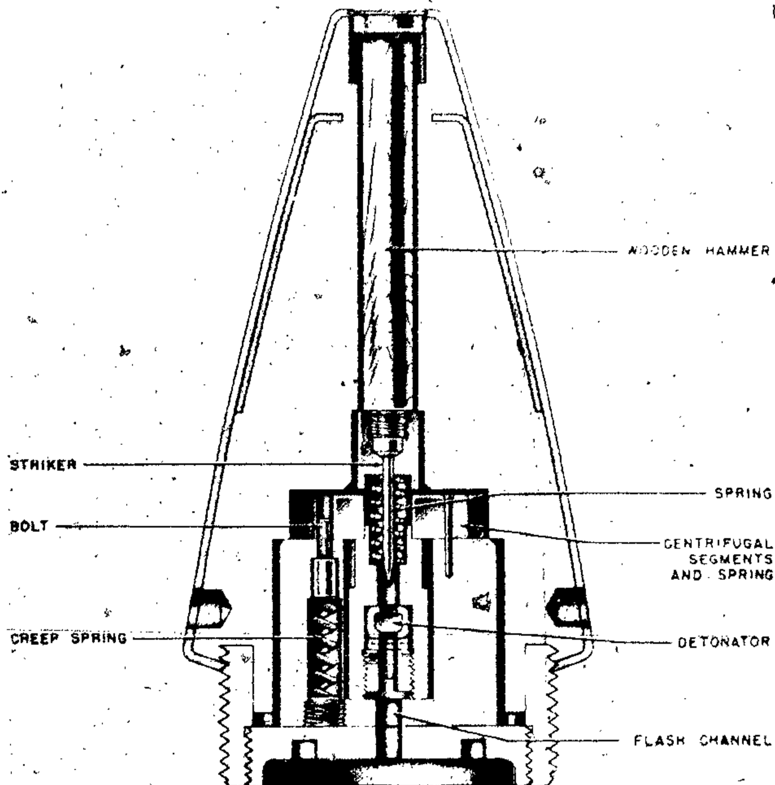
Figure 598—A. Z. 23 NB (Prebstoff)
