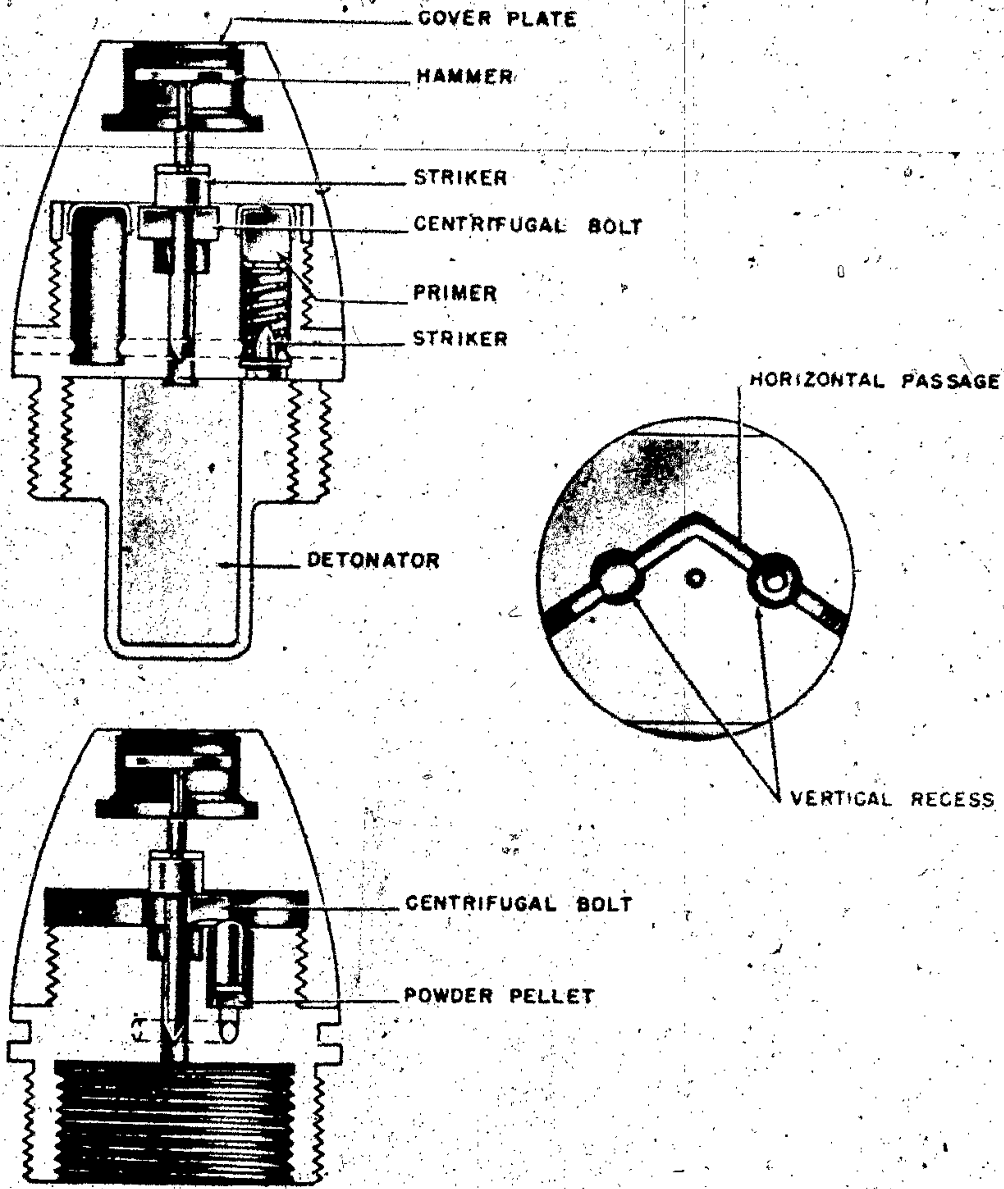
Figure 569—A. Z. 150 Rh. S.
