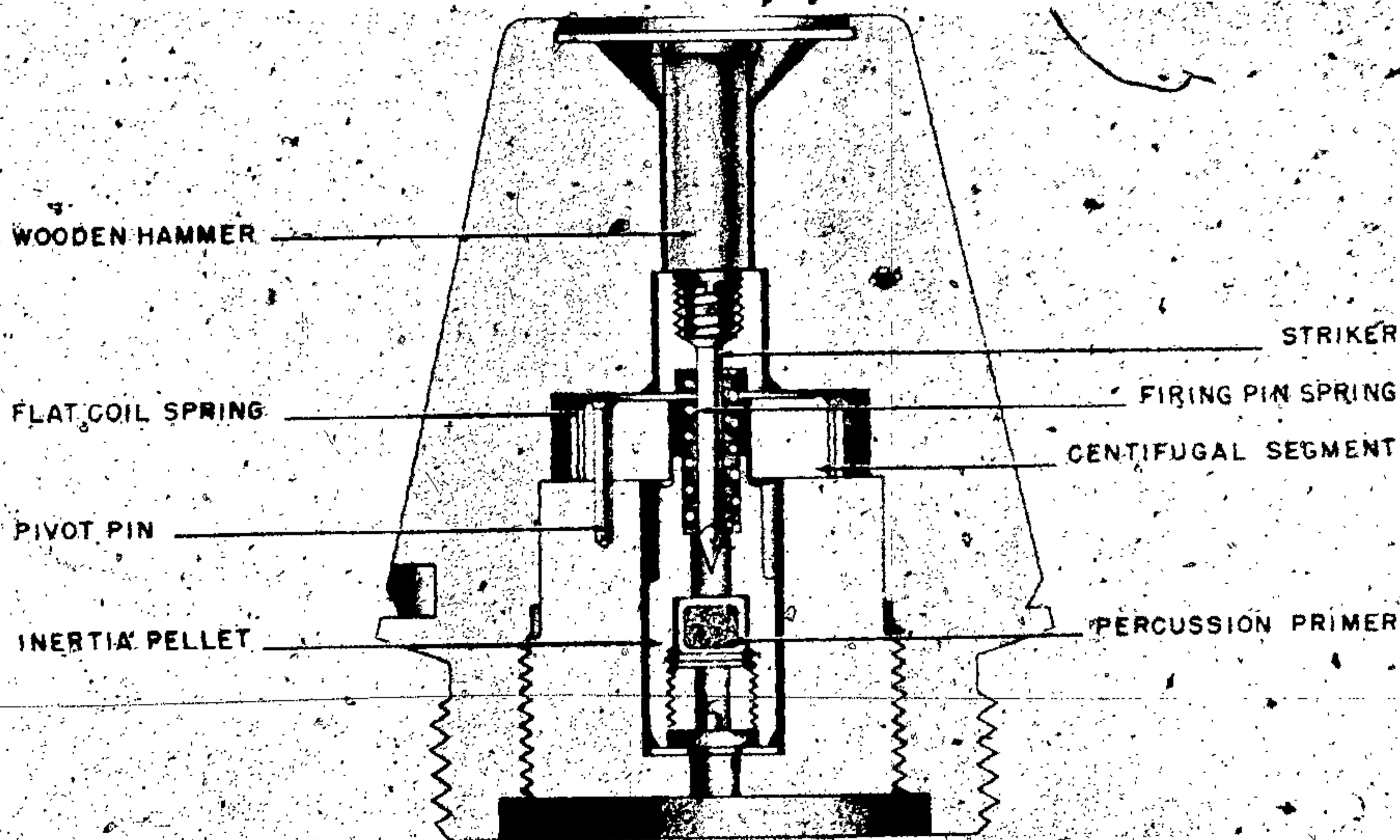
Figure 586—A. Z. f. Hbgr.
