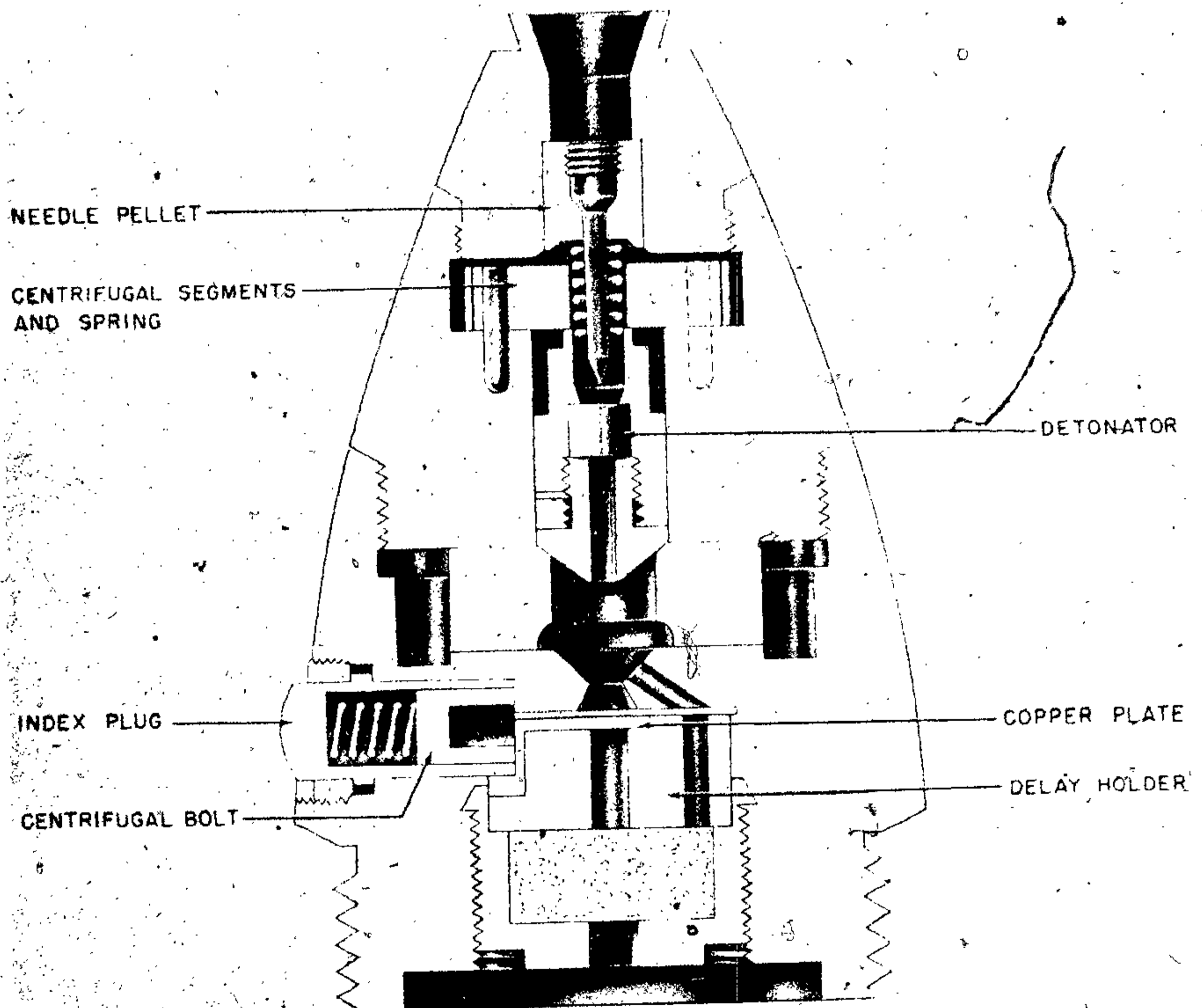
Figure 584—L. Jgr. Z 23 n. A.
