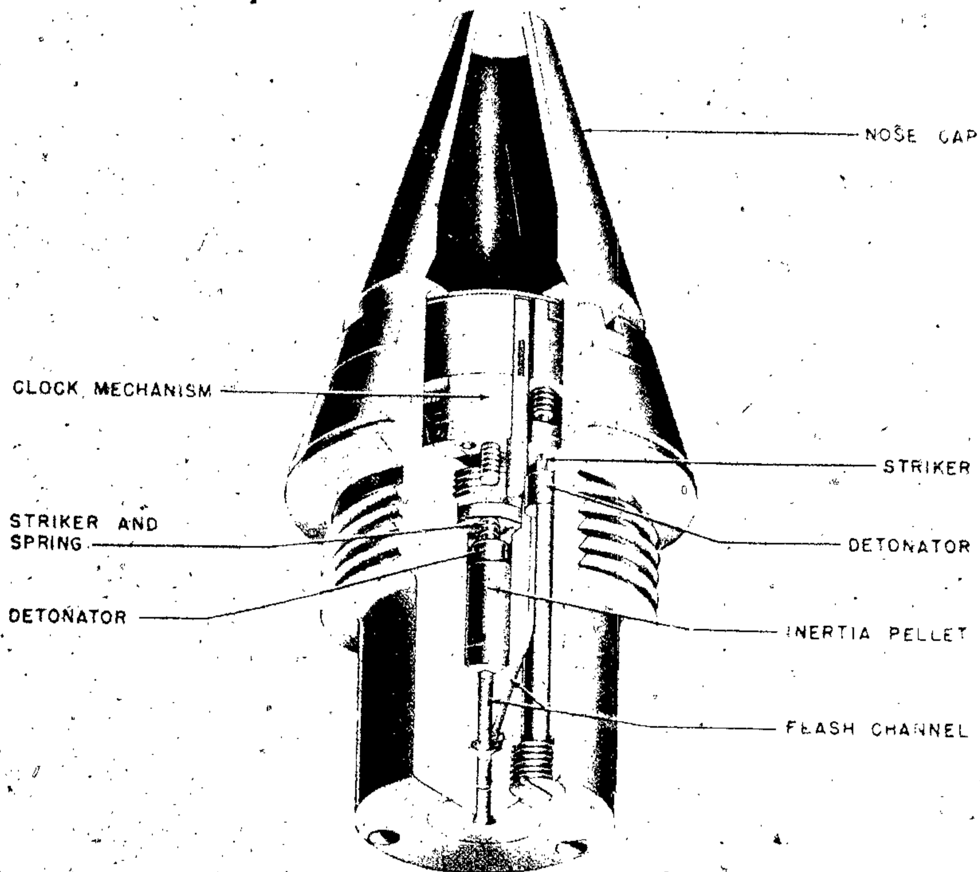
Figure 595B—Dopp. Z. 28 K
