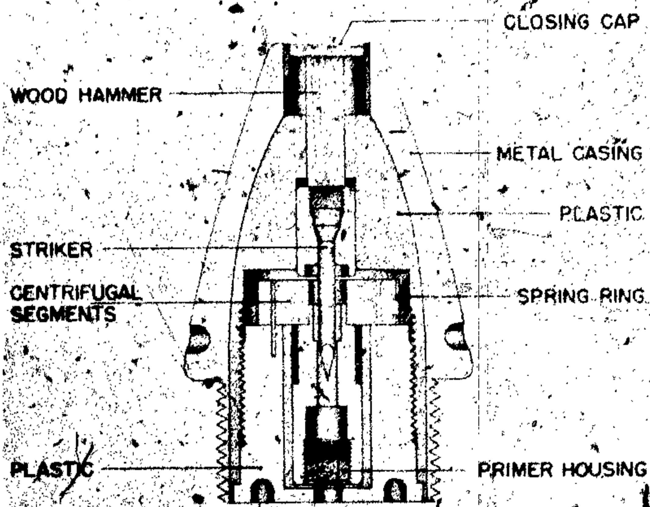
Figure 580—KI. A. Z. 23
