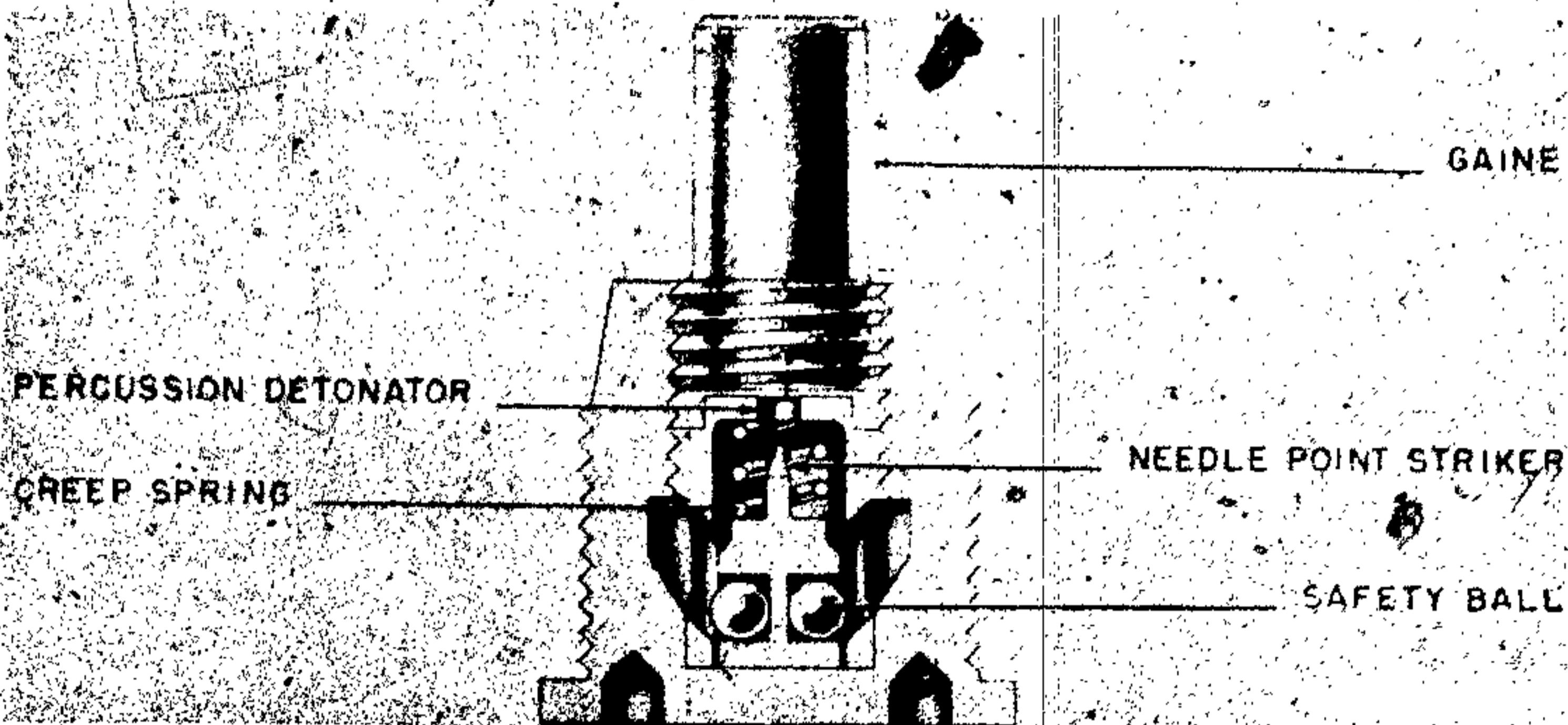
Figure 602—Skoda B. Z. 15-28-39
