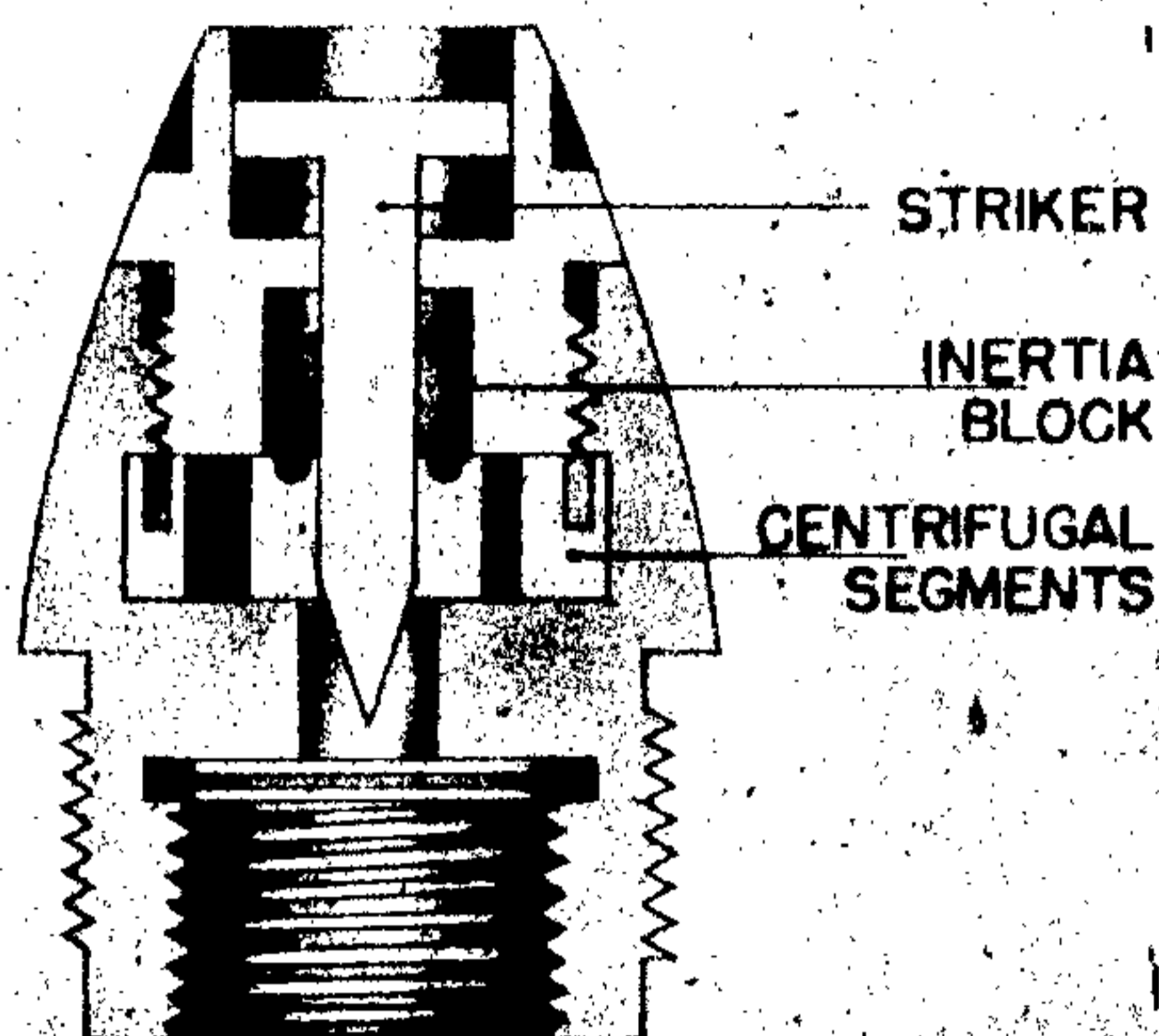
Figure 552—A. Z. 1502 F
