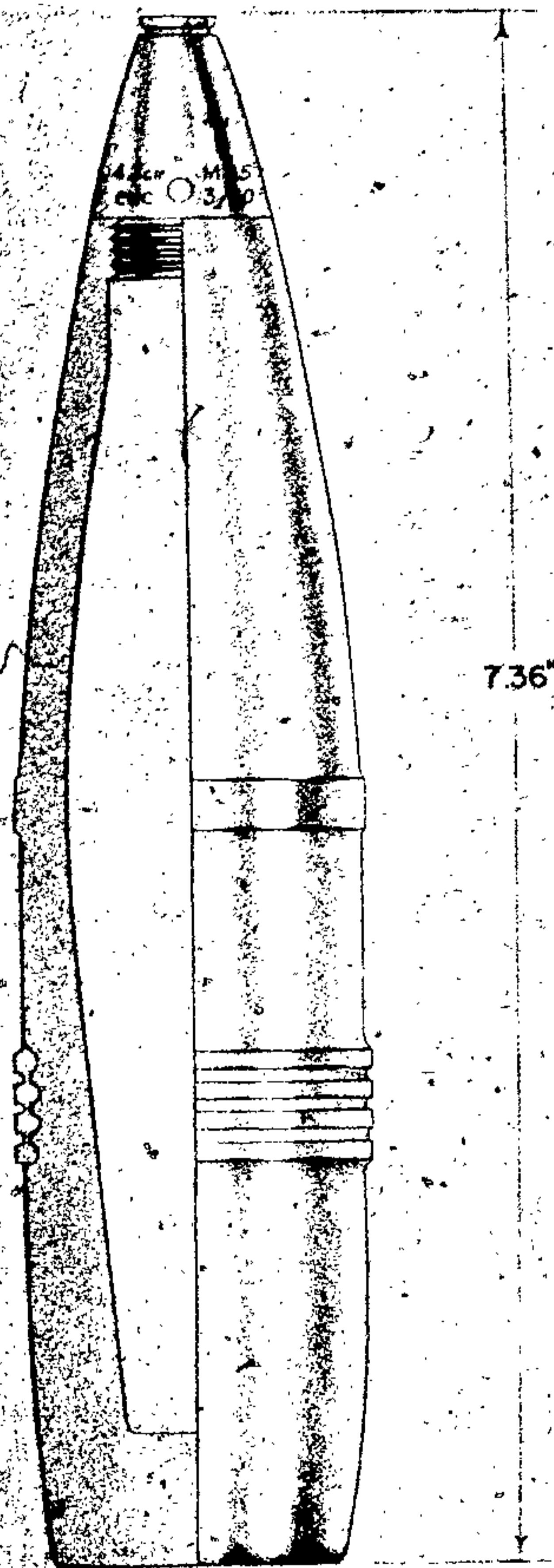
Figure 363—H. E. Projectile for Böhler Gun (Austrian Design) 47-mm, 4.7-cm Sprgr. Patr. (ö)
