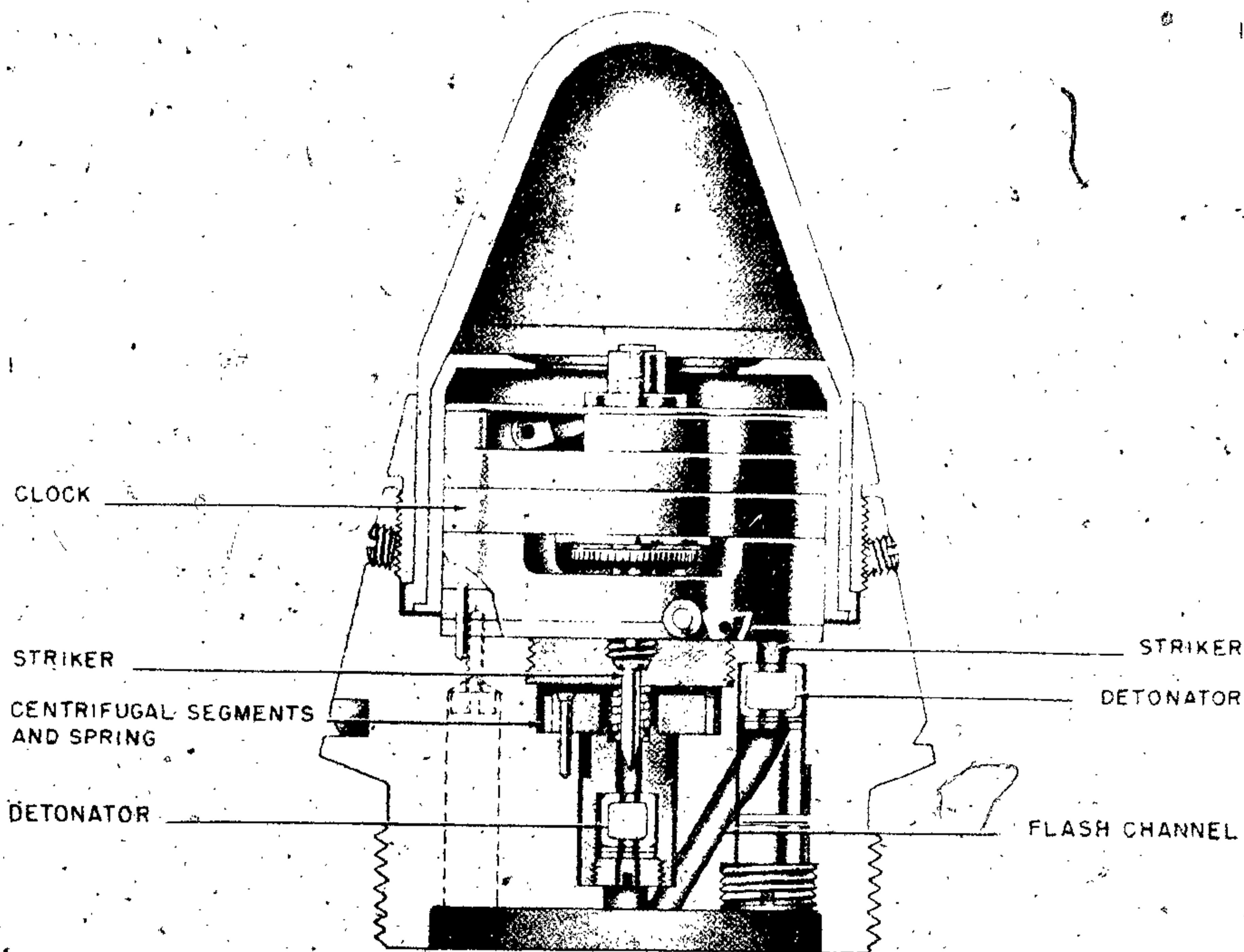
Figure 593C—Dopp. Z.S./160 Geb
