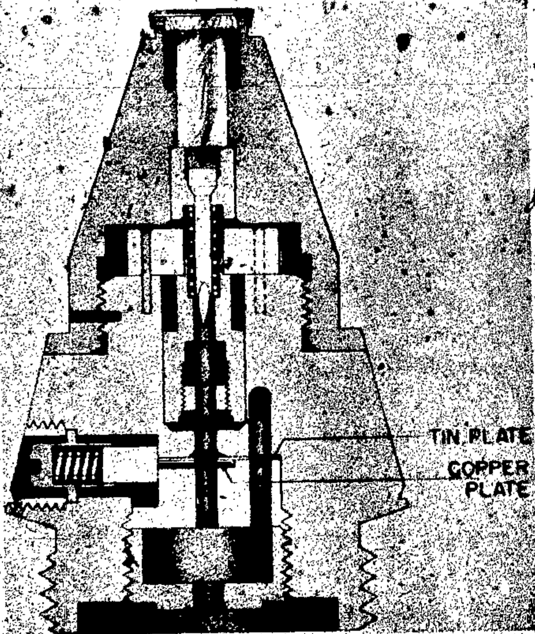
Figure 579—A. Z. 23 GEB
