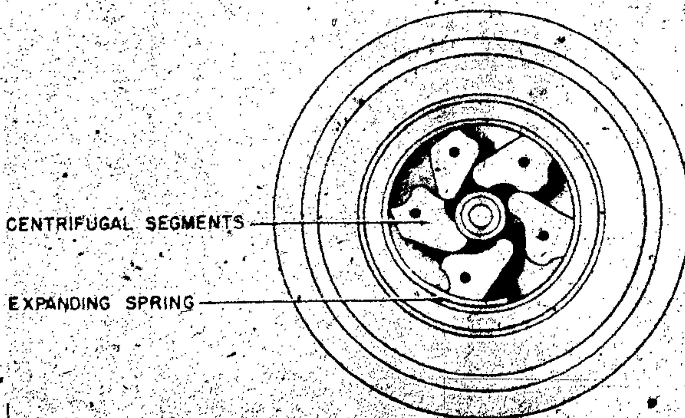
Figure 603—Bd. Z. C/38
