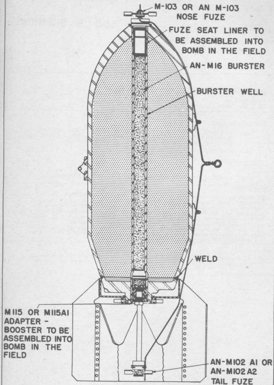
U. S. 1000 LB. CHEMICAL BOMB AN-M79
