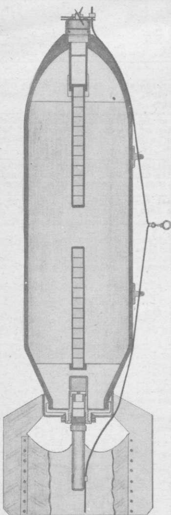
M32 600 LB.
