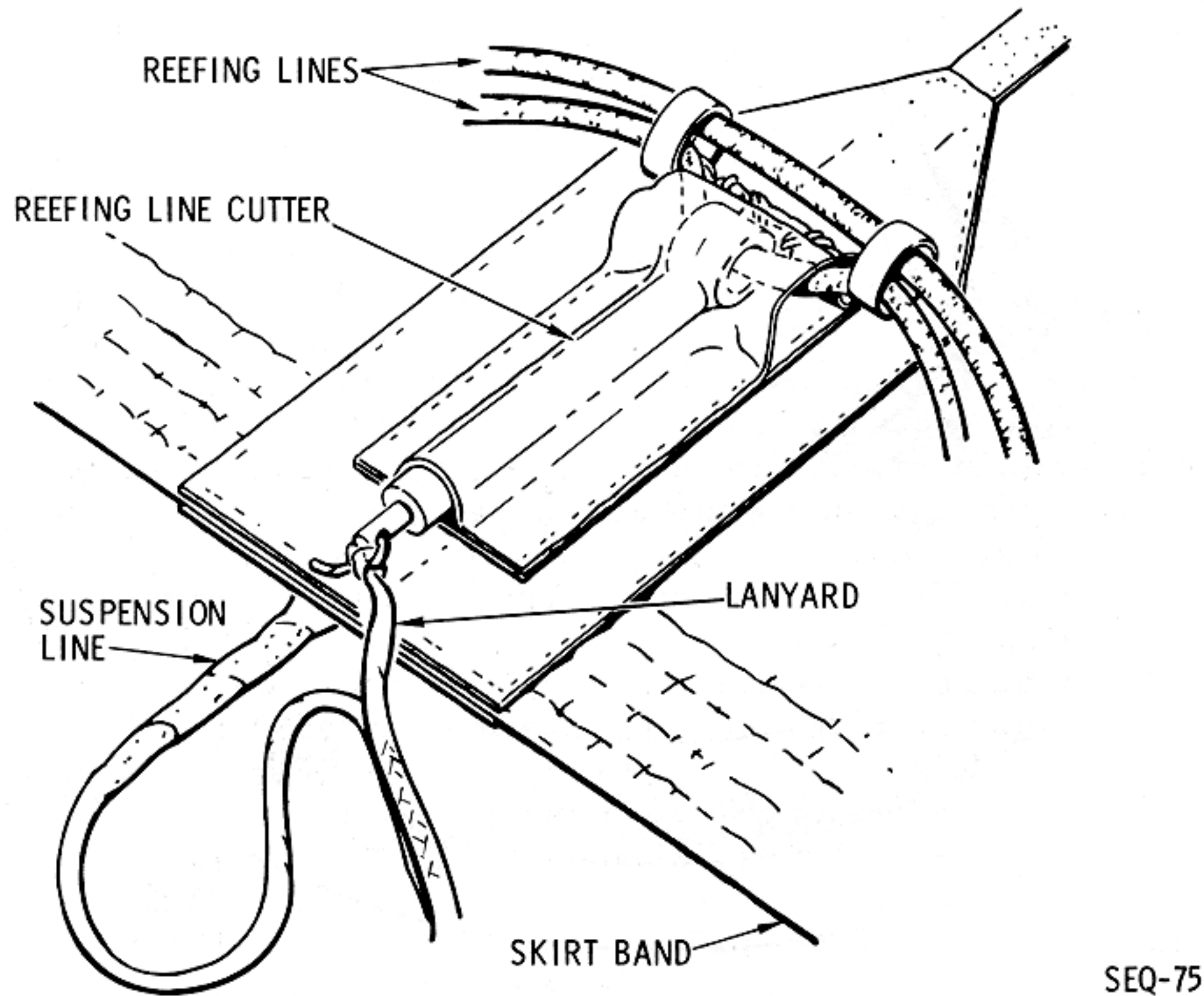
Figure 2.9-15. ELS Parachutes
