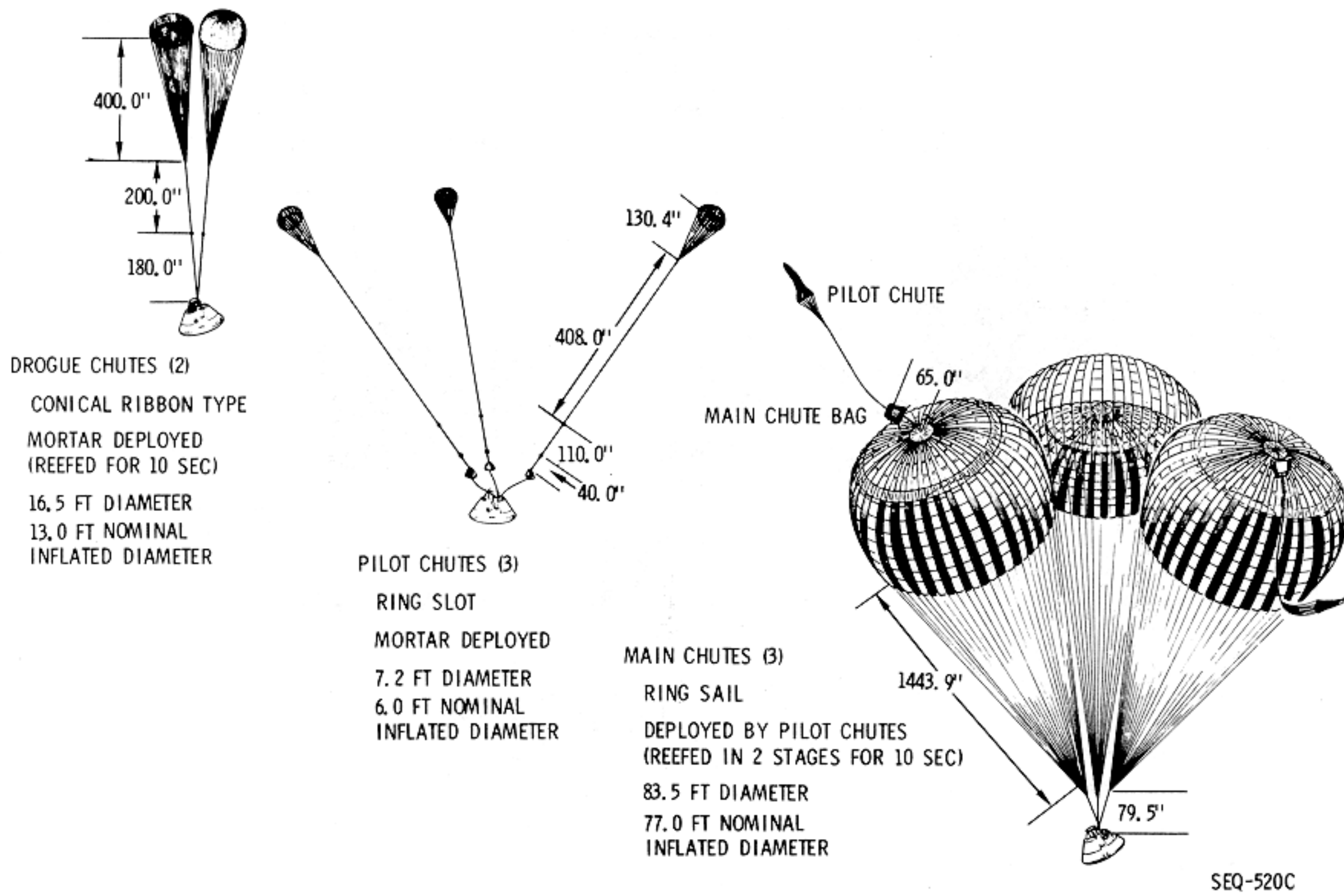
Figure 2.9-15. ELS Parachutes
