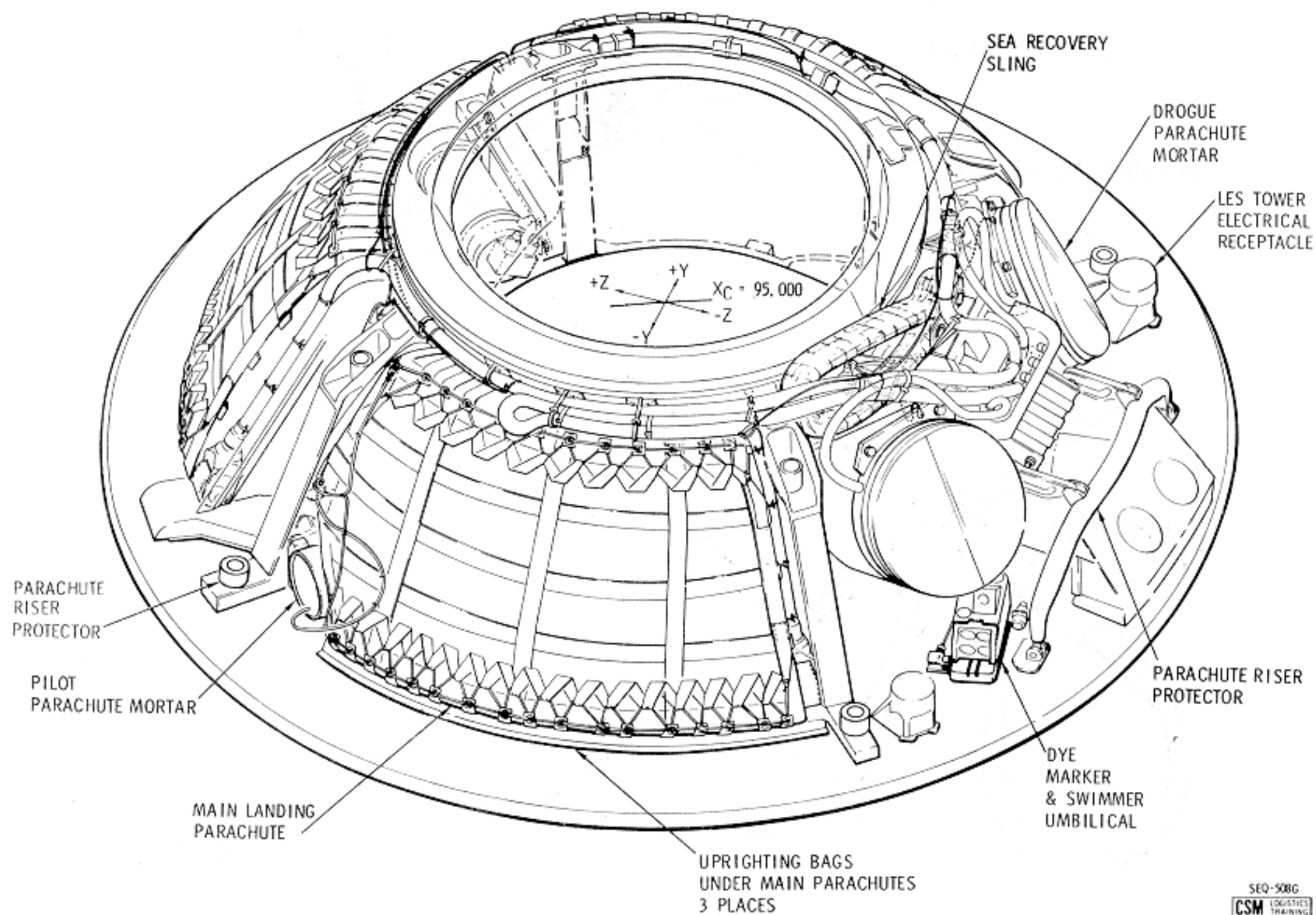
Figure 2.9-14. ELS Equipment
