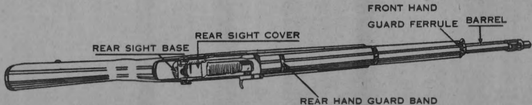
FIGURE 1.—U. S. rifle, caliber .30, M1.
