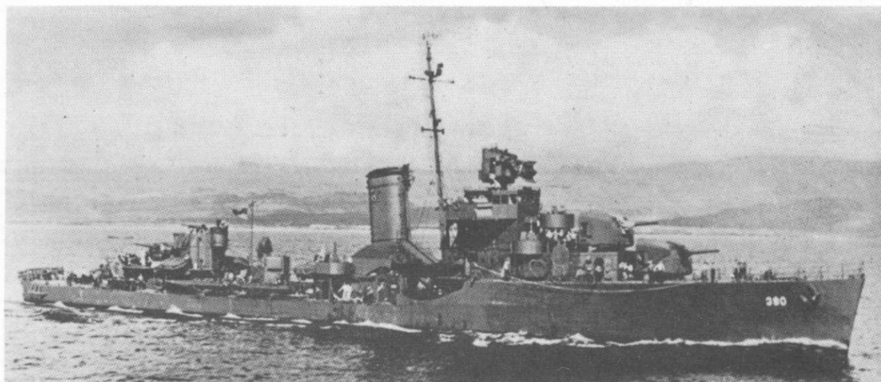
U. S. S. RALPH TALBOT (DD-390) (Bagley Class)
