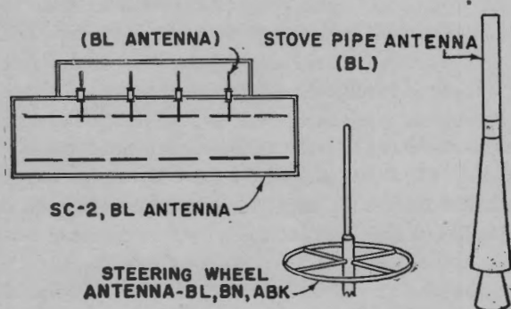
Figure 2-1. IFF antennas.
