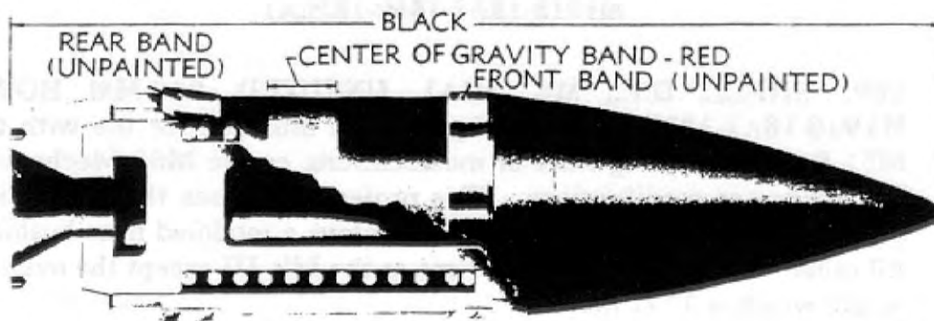
Figure 148 - PROJECTILE, Dummy, 360-lb., M12, 240-mm How., M1918-18A1-18MI-18MIA1, and M1
