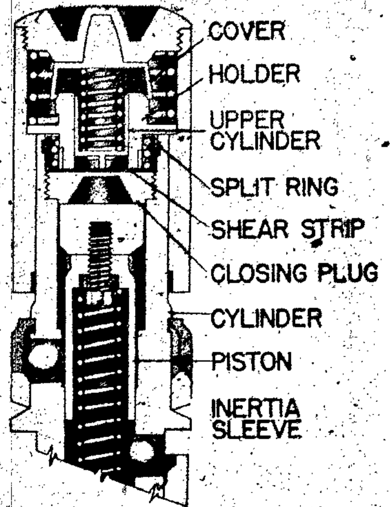
Figure 71 - "Manzolini", Fuze
