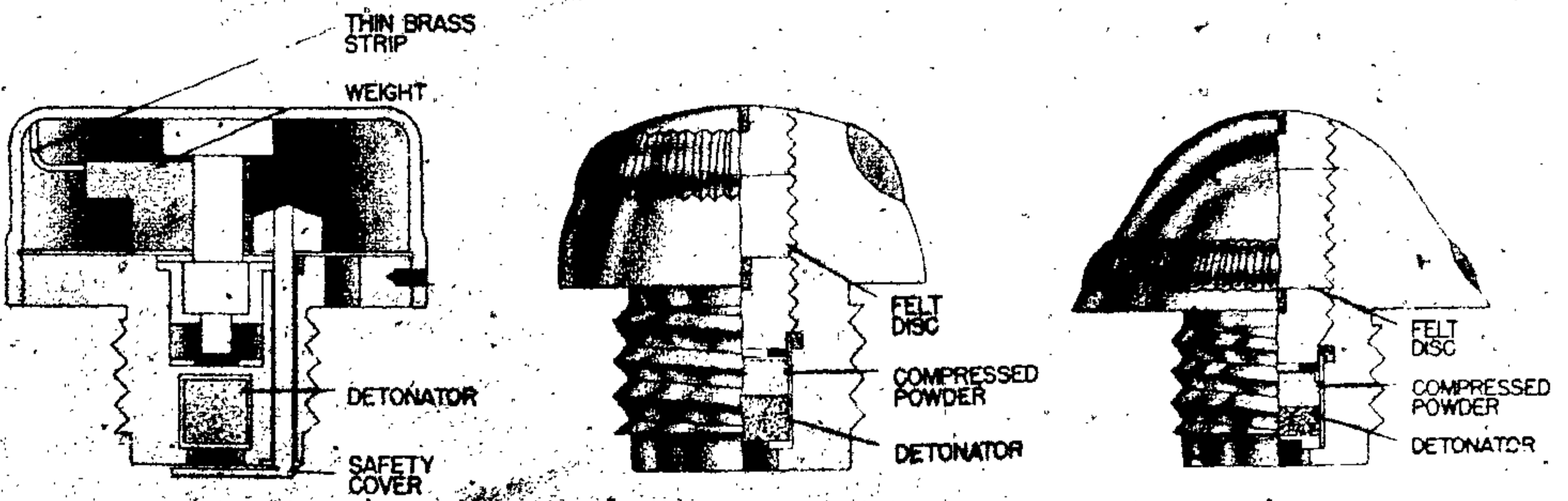
Figure 198 - Detonator M Cortese · Figure 199 - Detonator M10 (Allegenti) · Figure 200 - Detonator M10 (Allegenti)
