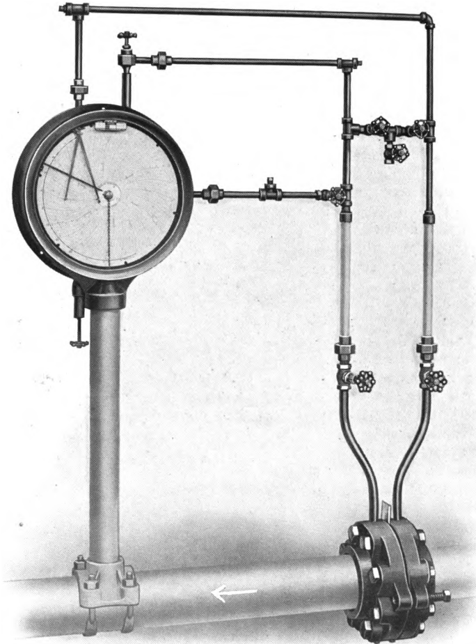
FIG. 1662. TYPE C METER
